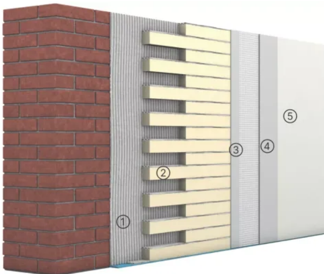
iQ-Therm 2.0 Systemaufbau
