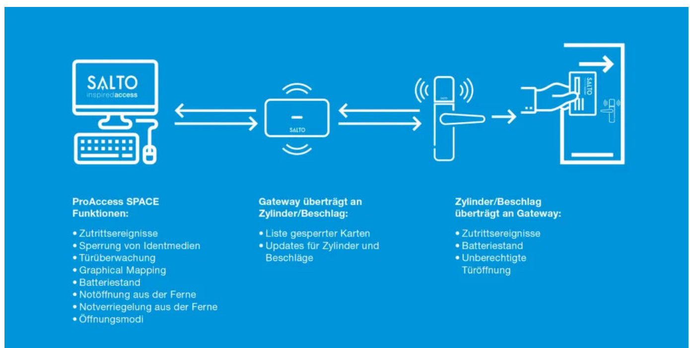
Salto BLUEnet - Kabellose Echtzeit Funkvernetzung
