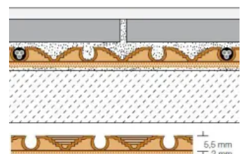
Schnittdarstellung Fußbodenaufbau: Schlüter®-DITRA-HEAT-DUO
