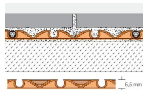
Schnittdarstellung Fußbodenaufbau: Schlüter®-DITRA-HEAT-E benötigt nur 5,5 mm zusätzliche Aufbauhöhe
