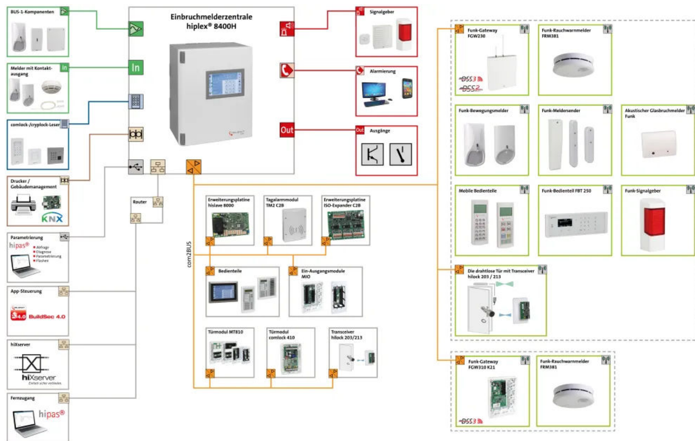
Übersichtsgrafik Gefahrenmeldeanlage © TELENOT
