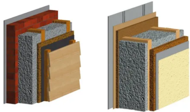
Fassadendämmung bei hinterlüfteter Fassadenbekleidung
