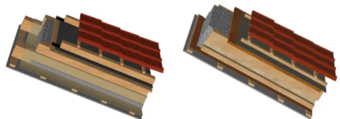
Dachdämmung von außen
