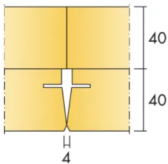
Systemskizze
