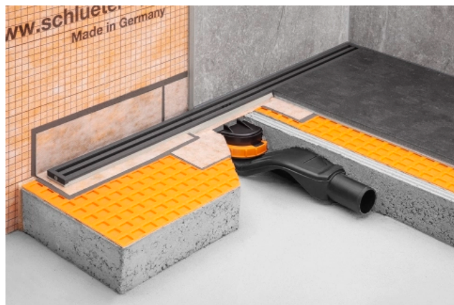
Linienentwässerung variabel neu gedacht
