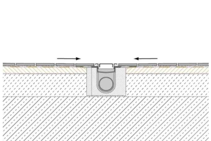
Einbauvariante Gefälleboard Mittelversion
