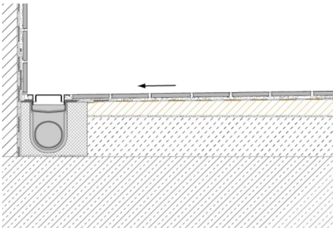
Einbauvariante Gefälleboard Wandversion
