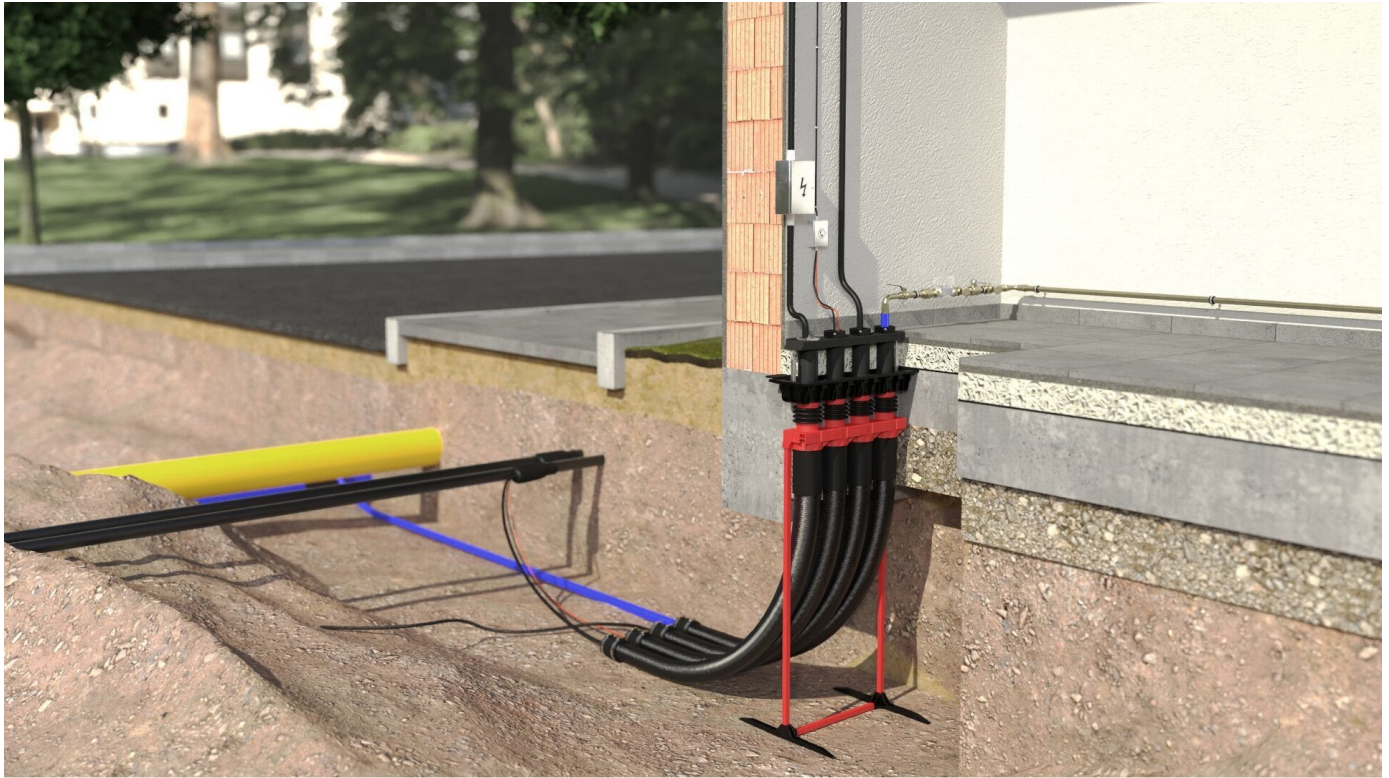
Das KRASO Bauherren-Komfortpakete: Mehrsparten-Hauseinführungen für Gas, Nah-/ Fern-/ Erdwärme, Wasser, Strom und Telekommunikation
