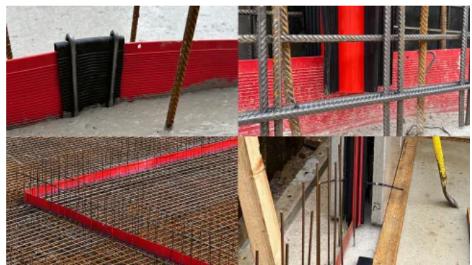
Fugenband und Fugenblech, Sternrohr
