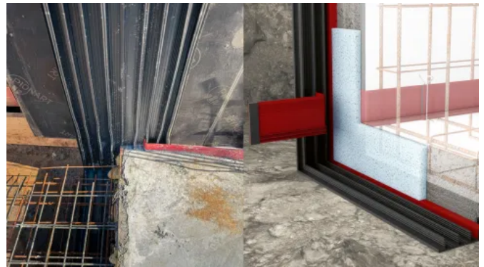
Systemfugenbänder
