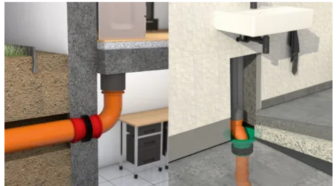
Boden- und Wanddurchführungen
