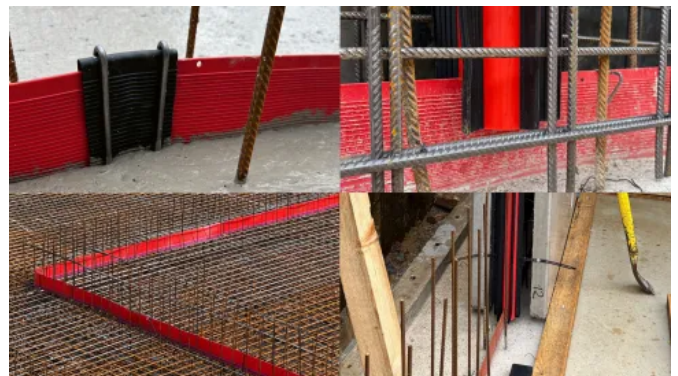
Fugenband und Fugenblech, Sternrohr
