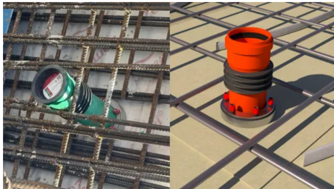
KRASO Bodendurchführung Typ FBV-BDF
