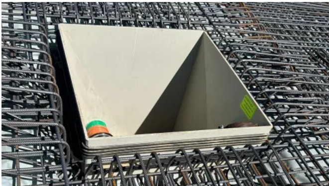
Pumpensumpf aus Kunststoff, eckig
