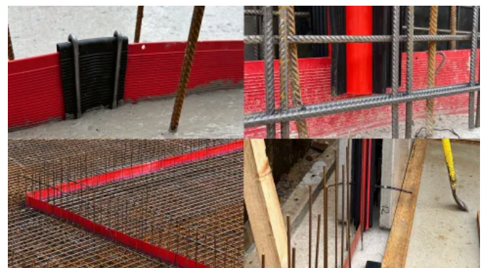
Fugenband und Fugenblech, Sternrohr
