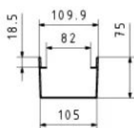
WOLFA Drainage Rinne Fixo 110
