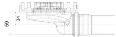
Seitlicher Ablaufanschluss mit Ablaufanschlussring NW 50
