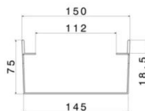
WOLFA Drainage Rinne Fixo 150
