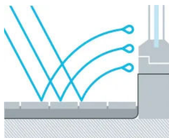
Ohne SitaDrain®: Gebäudeverschmutzung durch Wasser und Spritzregen.
