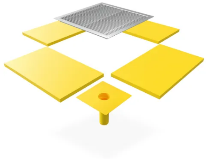
SitaDrain® Flächenrahmen
