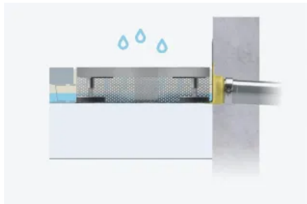
Mit optimal höhenverstellbaren FüÙen: SitaDrain® Terra
