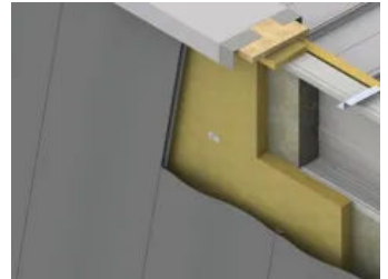
Oberer Fassadenabschluss – schräg auf Kassetten-Innenschale mit vorgesetzter Dämmung
