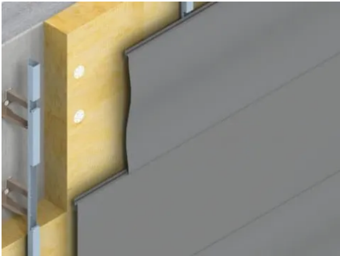
Hinterlüftete Fassade – waagrecht auf Betonwand mit Dämmung
