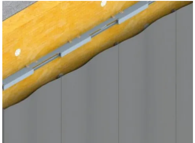
Hinterlüftete Fassade – senkrecht auf Betonwand mit Dämmung
