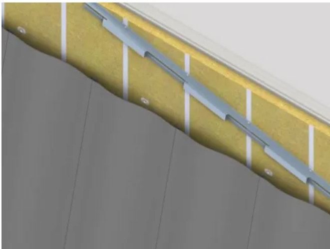
Hinterlüftete Fassade – schräg auf Kassetten-Innenschale mit vorgesetzter Dämmung
