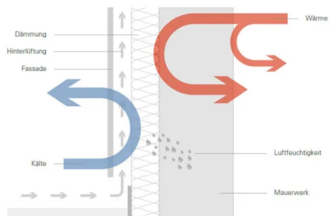
Konstruktion der vorgehängten hinterlüfteten Fassade (VHF)
