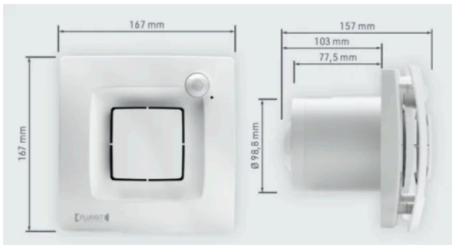
Dezentrales Abluftsystem Kwait 100 IQ
