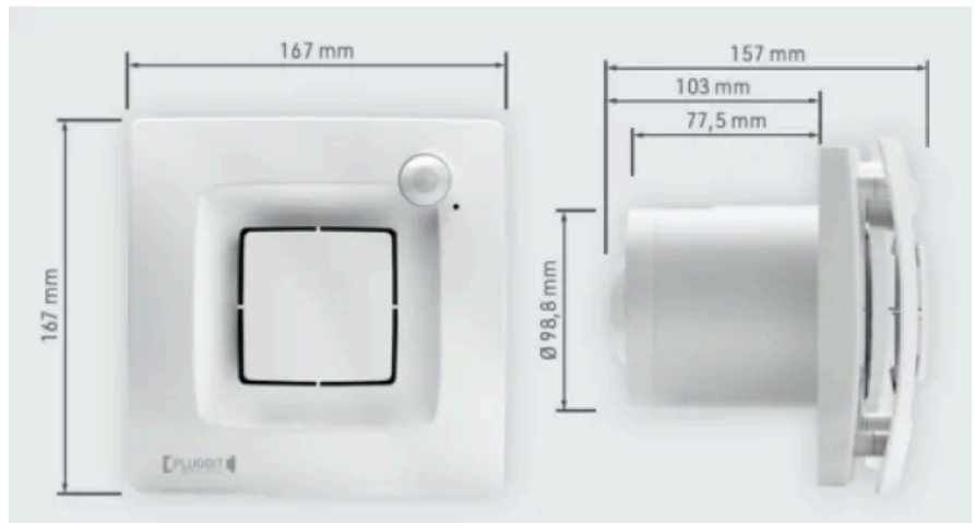
Dezentrales Abluftsystem Kwait 100 IQ
