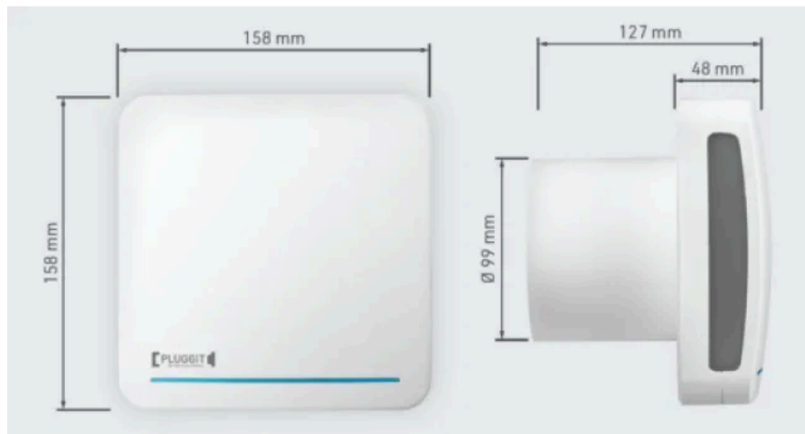
Zentrales Abluftsystem Kwait 100 PWR
