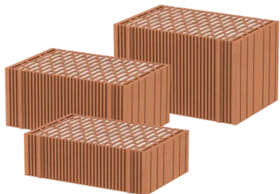
POROTON®-HAZ Höhenausgleichsziegel in den Höhen 11,5, 16,0 und 22,0 cm
