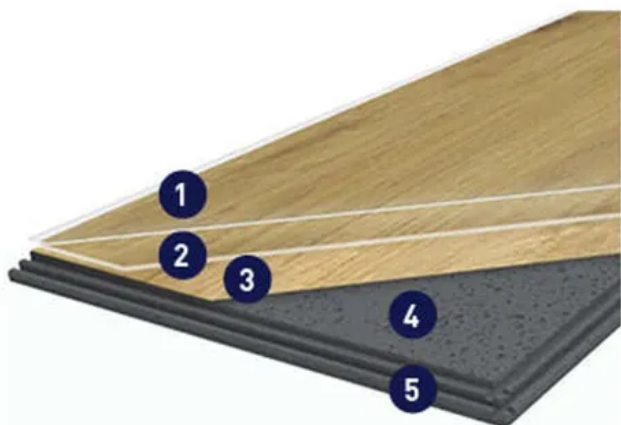
Vinyl-Objektfliesen CREATION 70 MEGACLIC | Produktaufbau
