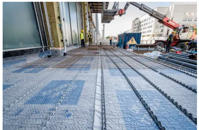
Mit DELTA®-TERRAXX lassen sich durch das Rollenformat 30 m 2 in einem Arbeitsgang schnell verlegen. (© Photo: Martin Matula Photography)
