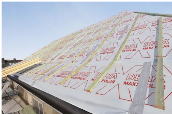
DELTA®-MAXX POLAR AL mit aufkaschierter Unterdeckbahn
