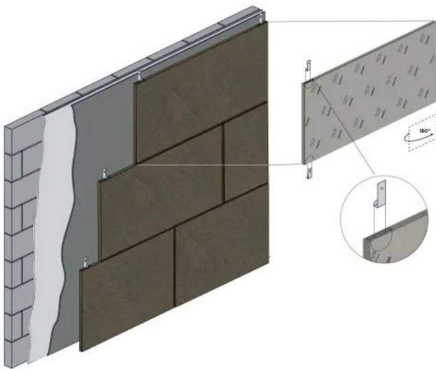
Systemskizze DKB
