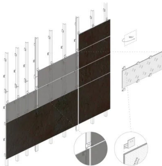
Systemskizze DKT3
