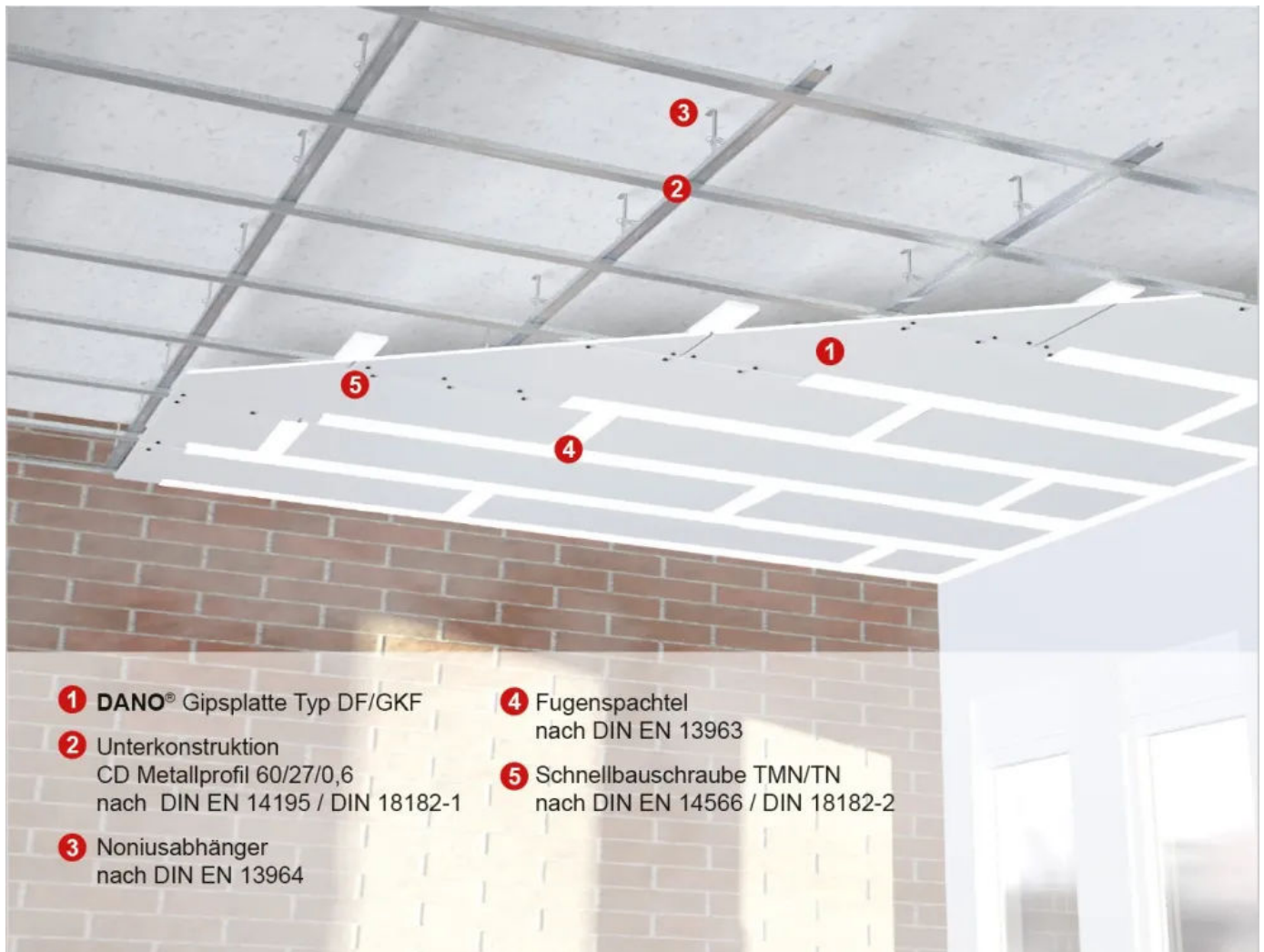
D 30-58 Unterdeckenbekleidung F30-A (1 x 20 mm Dano® Massiv DF/GKF)
