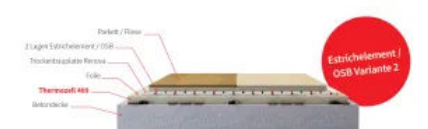
Thermozell mit Trockenestrich auf Betondecke
