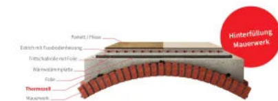
Thermozell für Mauerwerks-Hinterfüllung
