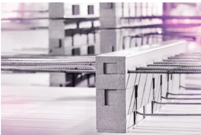
ISOPRO® Wärmedämmelement
