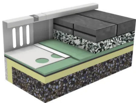
Kiesfangleiste - TYP F komplett
