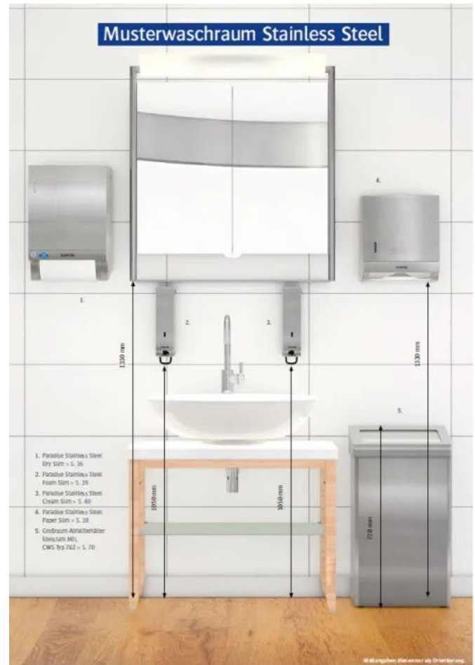
Musterwaschraum Stainless Steel mit optimaler Ausstattung und vorgeschlagenen Montagemaßen.
