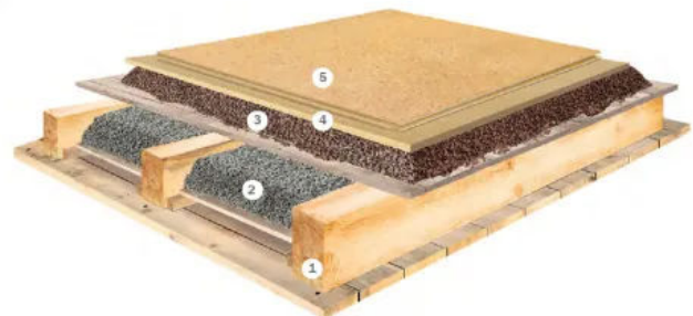
CW1000 Hohlraumschüttung in Holzbalkendecken
