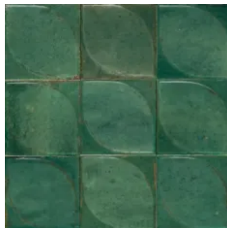
3D-Struktur Dew
