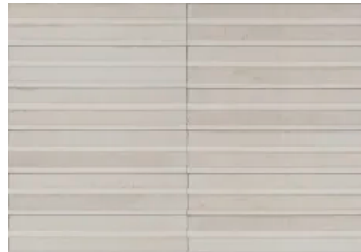
3D-Struktur Rake
