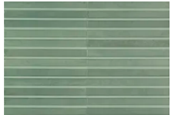
3D-Struktur Rake
