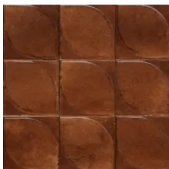
3D-Struktur Dew
