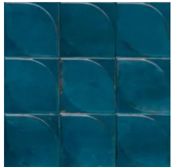
3D-Struktur Dew
