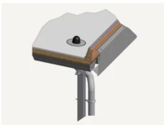
Dachtyp: Gründach
