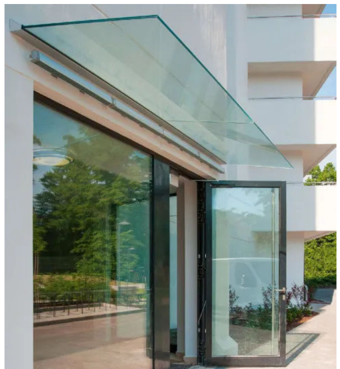
CANOPY cloud Lösung mit durchgehendem Profil und zwei aneinandergereihte Scheiben
