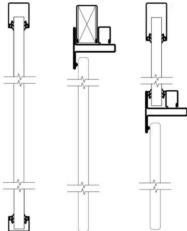
Vertikalschnitt Festwand Vertikalschnitte
