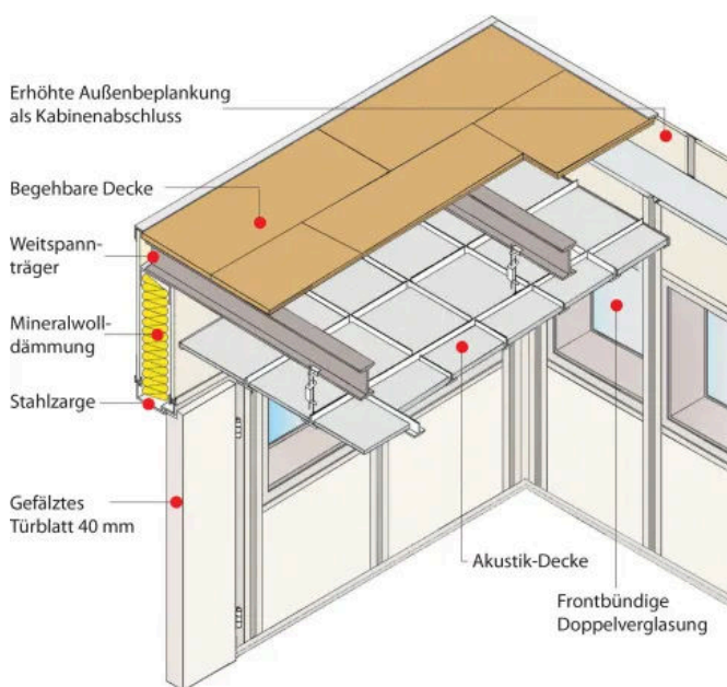
Doppelstock-Anlage, EG frei, OG 4-seitige Kabine
