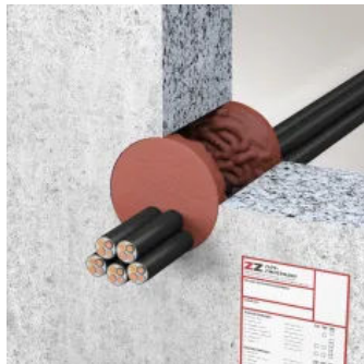
ZZ® C30-DE Kabelabschottung - Massivwand
