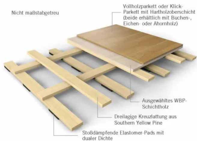
Harlequin WoodSpring Engineered Hardwood Top – mit Mehrschichtparkett – oder Solid Wood Top – mit Massivparkett
