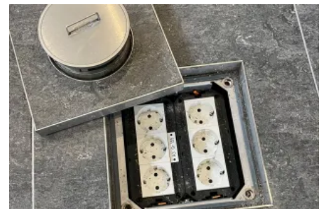
OKA-Kanäle ermöglichen den Einbau von Geräteeinsätzen für Steckdosen, Daten- und Multimediaanschlüsse (z.B. HDMI, USB).
