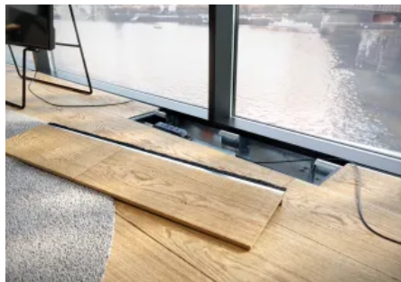
Fertig montierte OKB-Kanäle lassen sich auch nachträglich problemlos öffnen und mit Steckdosen, Daten- und Multimediaanschlüssen bestücken.
