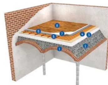
Systemskizze: Gewölbedämmung mit GEOMATERIALS Blähglas
