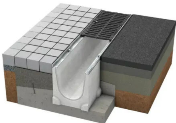
BIRCOlight® triloc®
