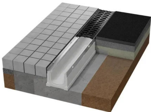
BIRCOslim®
