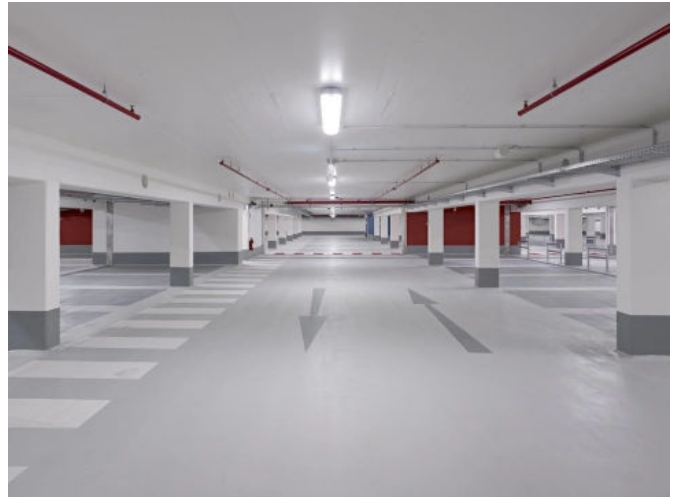
Sanierung mit Betoninstandsetzung, Wände und Stützensockel, Tiefgarage Platz D'Agen, Dinslaken. Foto: Guido Erbring
