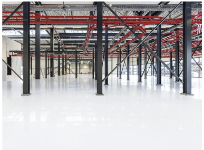
Chemikalienbeständiger Boden für Lackierhalle, Melle, DE. System: StoPox GH 530, StoPox KU 601. Foto: StoCretec
