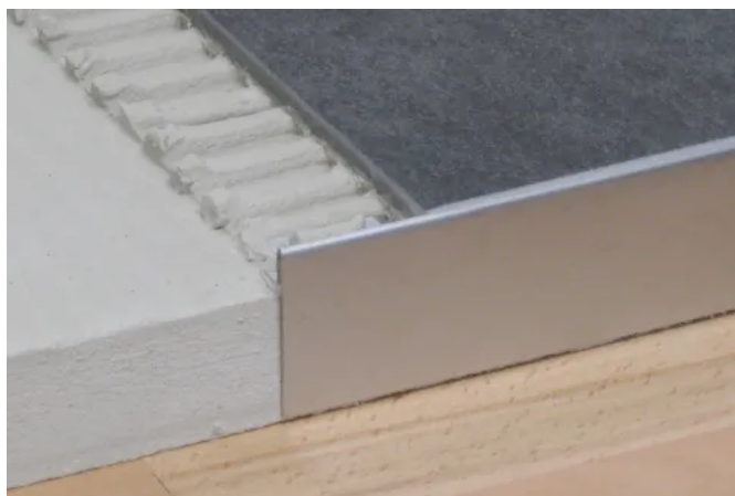
BLANKE SCHWELLENPROFIL
