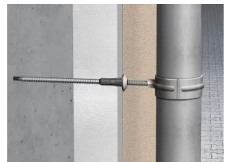
Würth AMO®-Therm Mini für Regenfallrohrbefestigung in einer Betonwand mit Dämmung
