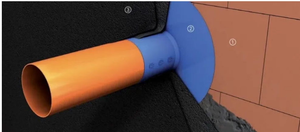
Rohrdurchführung in drei Schritten abdichten: (1) Untergrund reinigen und Rohr fixieren, (2) Flanschkleber auf Rohrflansch und Untergrund auftragen, (3) Rohrflansch um das Rohr setzen und die Bauwerksabdichtung mit MB-Produkten oder Remmers PMBCs anschließen.
