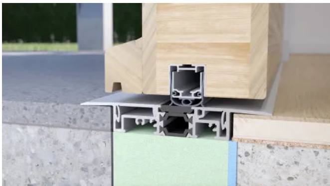
Um seine Energiespar- und Dichtleistungen noch weiter zu optimieren, lässt sich das Nullschwellen-Set Comfort-Plan® mit bauseitigen Unterbaudämmprofilen und Drainage-Lösungen kombinieren.
