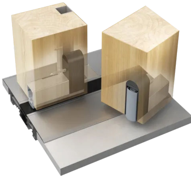
Schlagregendichte Dichtung für 2-flg. Türen mit universeller Einstellung im Mittelstulp
