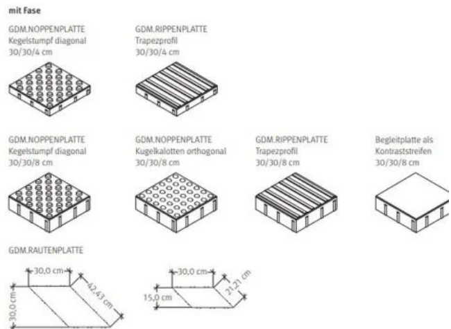
GDM.TAKTILE LEITSYSTEME
