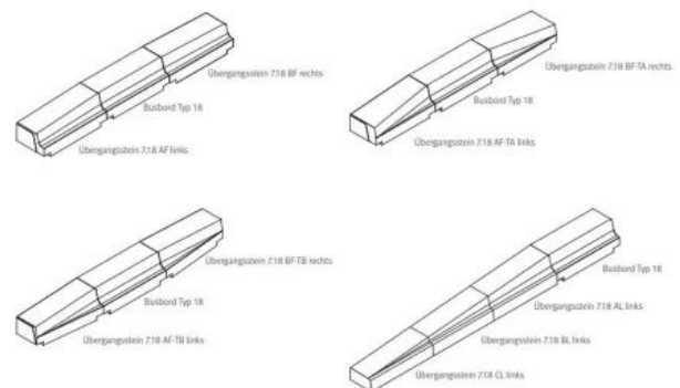
GDM.BUSBORD
