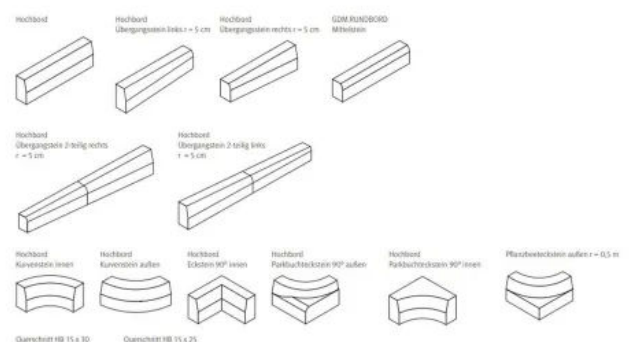
GDM.HOCHBORD
