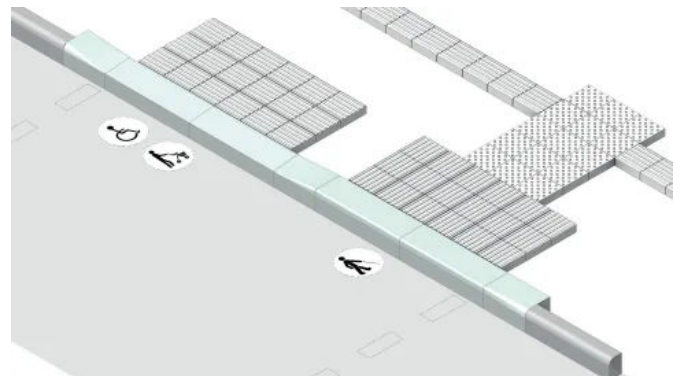
Beispiel für eine gesicherte Überquerungsstelle mit Bodenindikatoren nach DIN 32984
