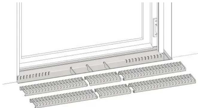
6-teilige Abdeckung zur problemlosen Entnahme, z. B. zum leichten Reinigen der Rinne
