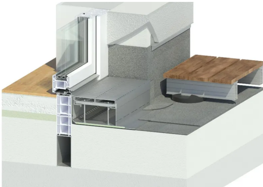
Barrierefreie Fassadenrinne INNORIN® F für den wärmebrückenfreien Anschluss an begehbare Flachdächern
