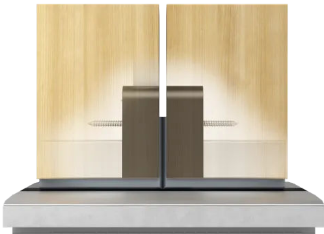
Rainstop® LC-17/20 WS mit universeller Einstellung im Mittelstulp
