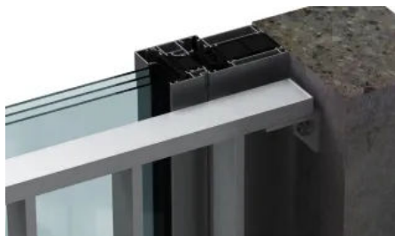
Befestigungsvariante in der Laibung
