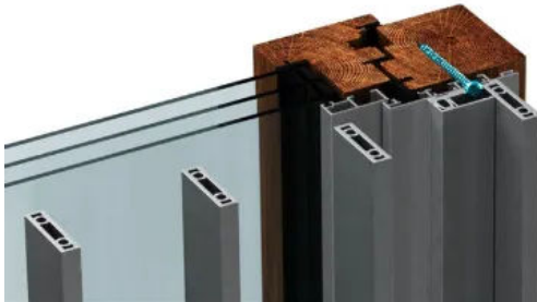
BALUGA easy balcony am Holz-Alu-Fenster
