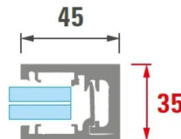
Systemschnitt
