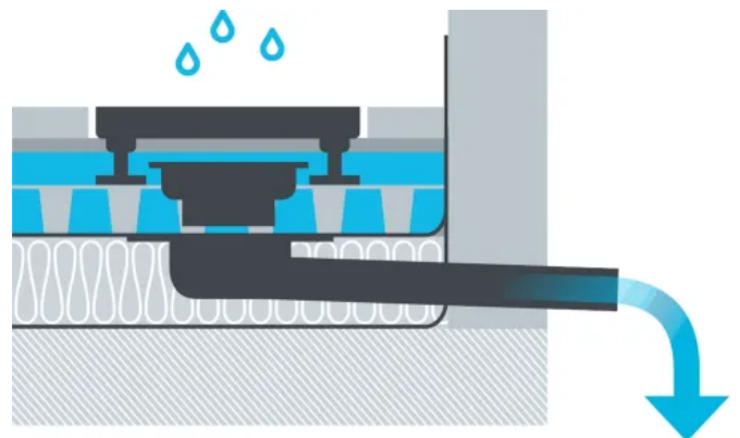
Dachgully abgewinkelt, mit Balkonaufsatz als Notentwässerung
