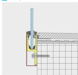
7 Anbindung seitlich an Balkon
