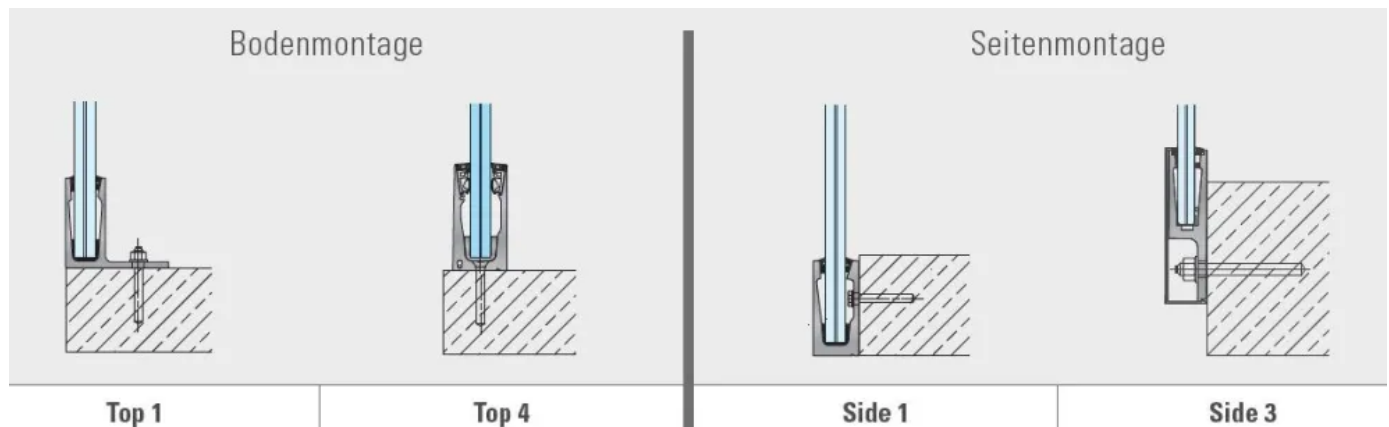
Profilübersicht BALARDO hybrid lite / hybrid / hybrid hd
