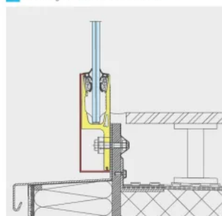
8 Anbindung seitlich mit hohem Fußboden
