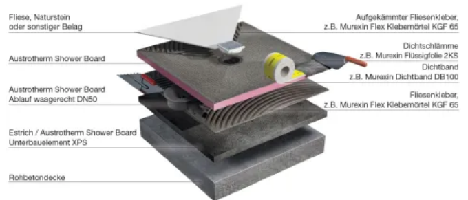
Bodenaufbau Austrotherm Shower Board
