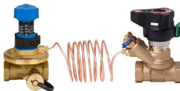
Automatische Strangventile, Set aus ASV-PV und ASV-BD
